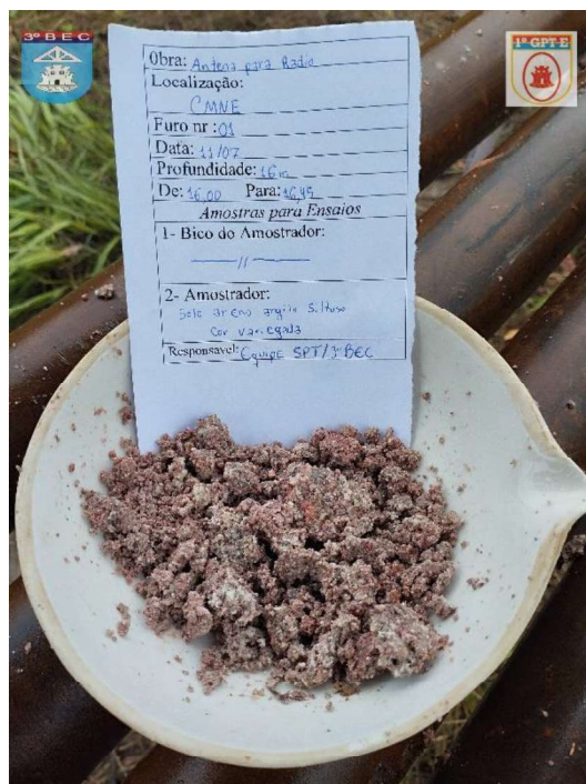
FURO 01 – PROF:16,00 PARA 16,45 SOLO ARENO ARGILO SILTOSO, COR VARIEGADO.
