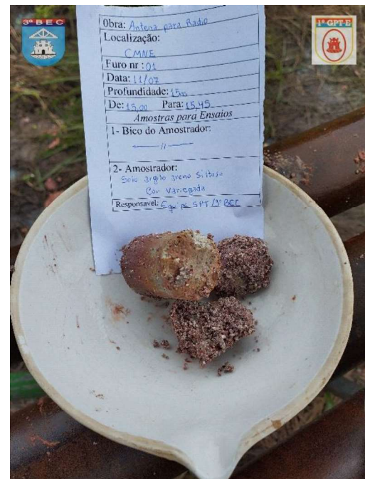
FURO 02 – PROF:15,00 PARA 15,45 - SOLO ARGILO ARENO SILTOSO, COR VARIEGADO.
