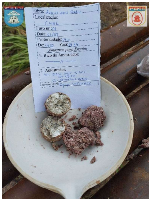
FURO 01 – PROF:14,00 PARA 14,45 - SOLO ARENO ARGILO SILTOSO COM SEIXOS, COR VERMELHA E BRANCA.
