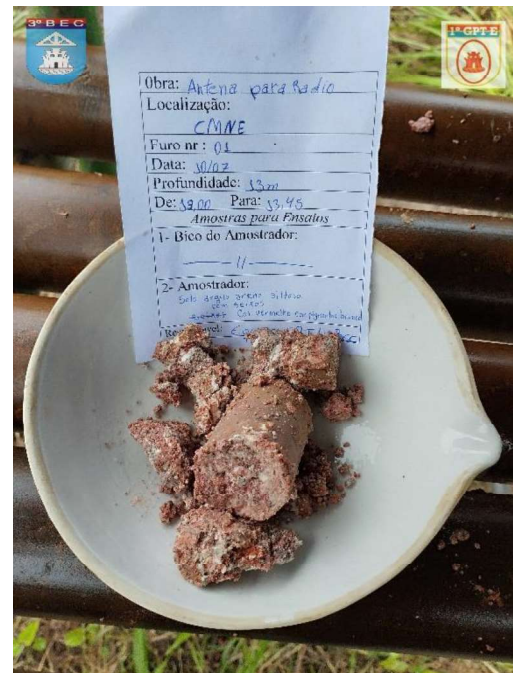
FURO 01 – PROF:13,00 PARA 13,45 - SOLO ARGILO ARENO SILTOSO, COM SEIXOS, CO VERMELHA.
